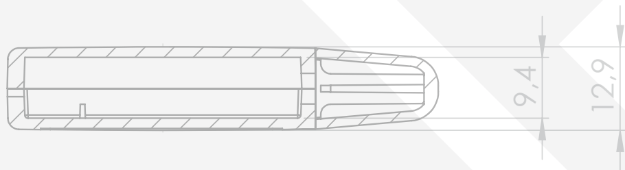
SECTION A-A
